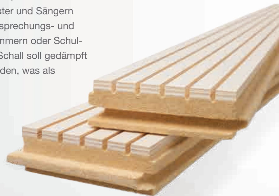
StudioLine Plus Akustikdecke
